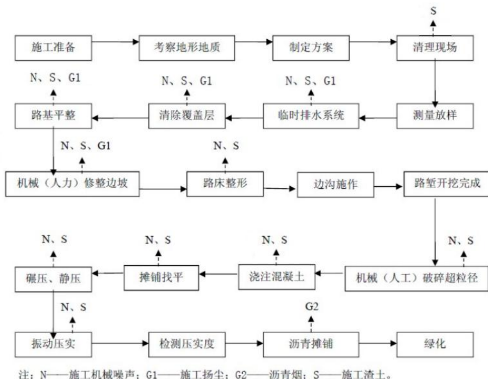
图 2-3 拟建项目道路工艺流程示意图
