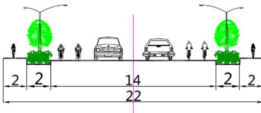
图 2-1 横塘浜路（龙锦路-后曹路）道路横断面图 单位：m
