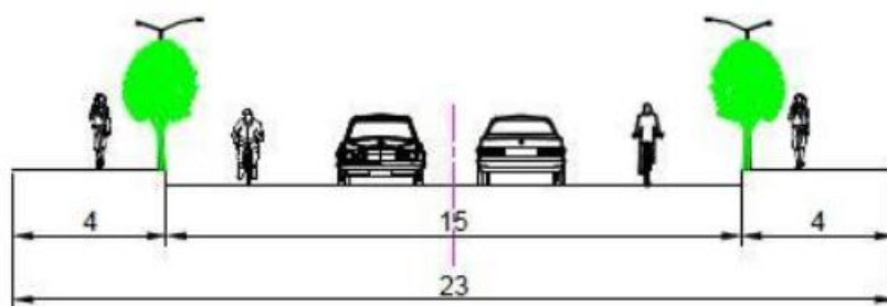
图 2-2 后曹路（紫林路-横塘浜路）道路横断面图 单位：m
