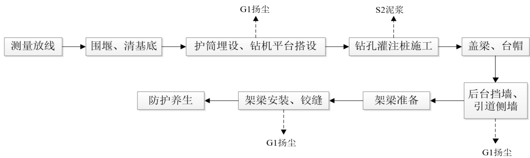
图 2-5 桥梁工程施工流程图及产污环节分析
